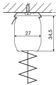
Motor-/Kettenzugprofil mit Deckenclip, 27 mm
