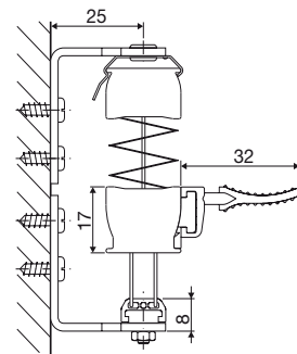
Gespannte Anlage mit Wandhalterbefestigung
