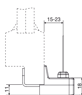
Seilbefestigung mit Klemmträger
