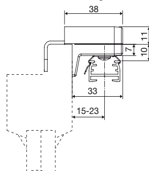
Standardprofil mit Klemmträger + Deckenclip
