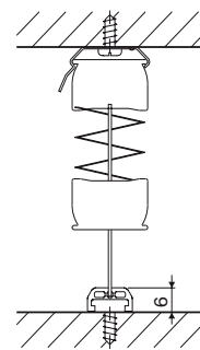
Gespannte Anlage mit Wandhalterbefestigung
