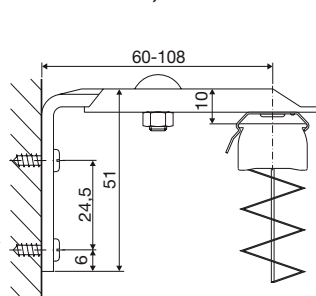
Standardprofil mit Wandhalter, 60-108 mm
