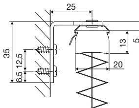
Standardprofil mit Wandhalter + Deckenclip
