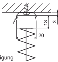
Standardprofil mit Deckenclip, 20 mm
