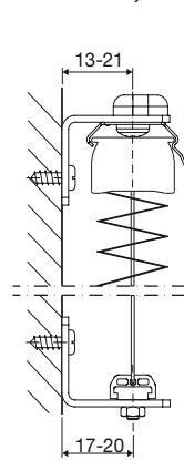
Seilbefestigung mit Klemmträger
